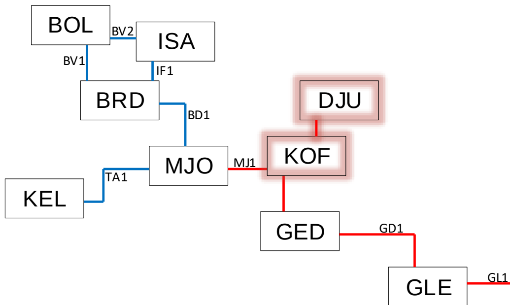
MYND 3-66 : AFHENDINGARSTAÐUR Í DJÚPI – EINLÍNUMYND AF FLUTNINGSKERFI VESTFJARÐA
