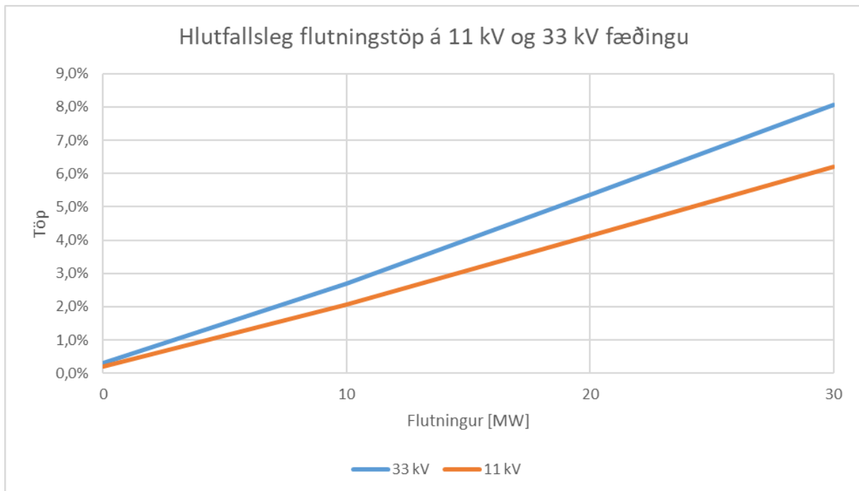
MYND 3-44 : HLUTFALLSLEG FLUTNINGSTÖP TIL HÚSAVÍKUR
