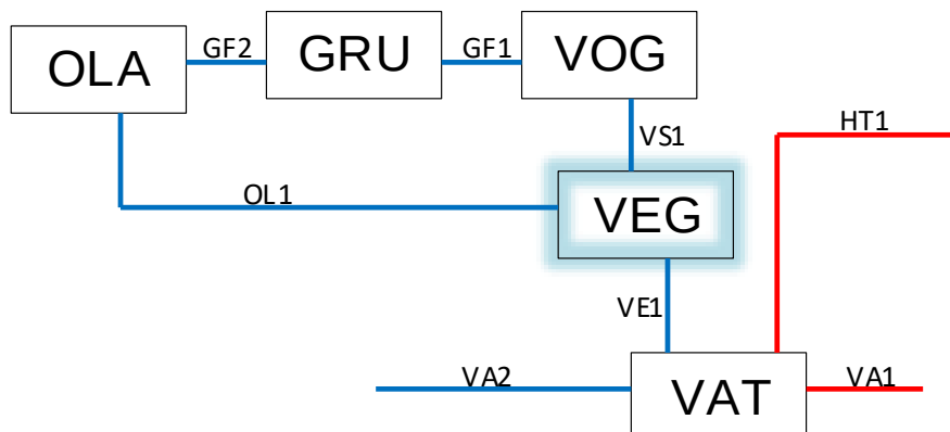
MYND 3-69 : VEGAMÓT – EINLÍNUMYND
