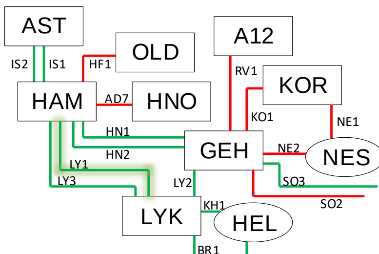
MYND 3-61 : YFIRLITSMYND LÍNULEIÐAR LYKLAFELLSLÍNU 1
