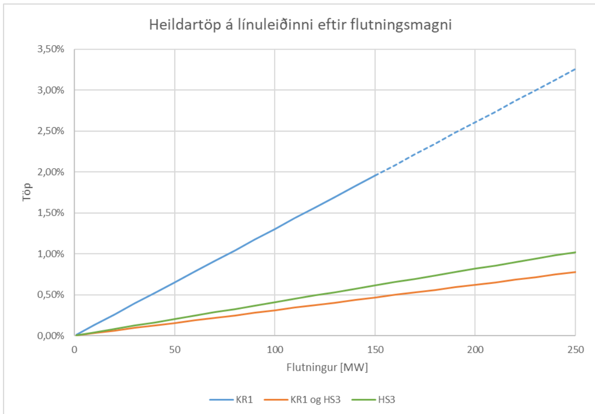
MYND 3-26 : HÓLASANDSLÍNA 3, FLUTNINGSTÖPIN SEM FALL AF FLUTTU AFLI
