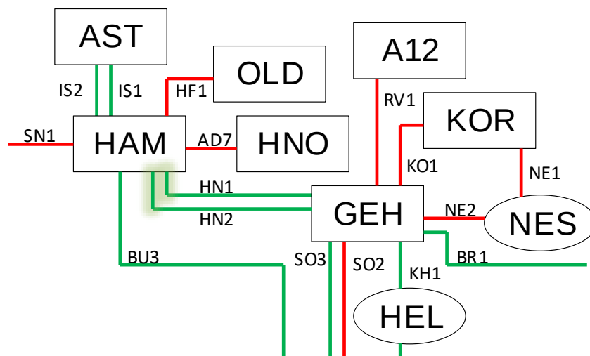
MYND 3-21 : HN1&amp;2 – EINLÍNUMYND
