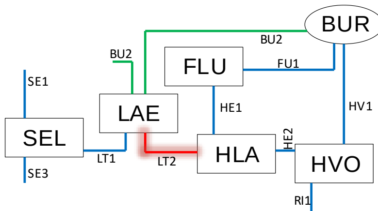
MYND 3-37. LT2 – EINLÍNUMYND MEÐ LÆKJARTÚNSLÍNU 2
