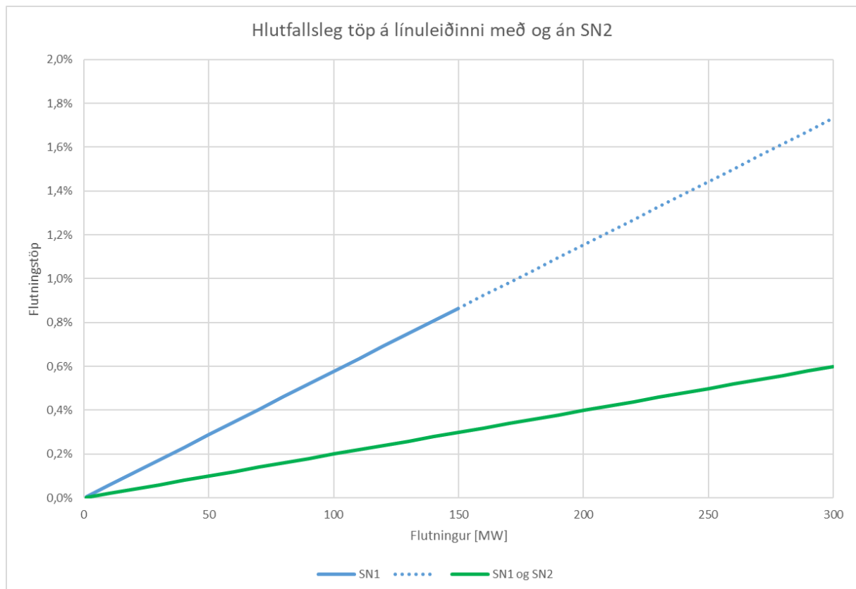
MYND 3-31 : HLUTFALLSLEG TÖP Á MILLI HAMRANESS OG FITJA
