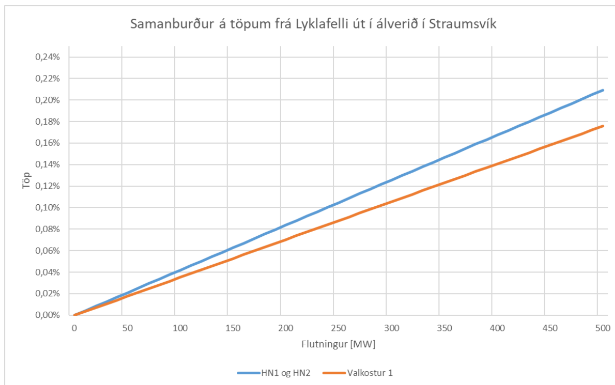
MYND 3-63 : SAMANBURÐUR Á HLUTFALLSLEGUM FLUTNINGSTÖPUM
