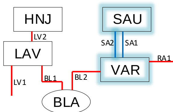
MYND 3-15 : EINLÍNUMYND SAUÐÁRKRÚKSLÍNU 2
