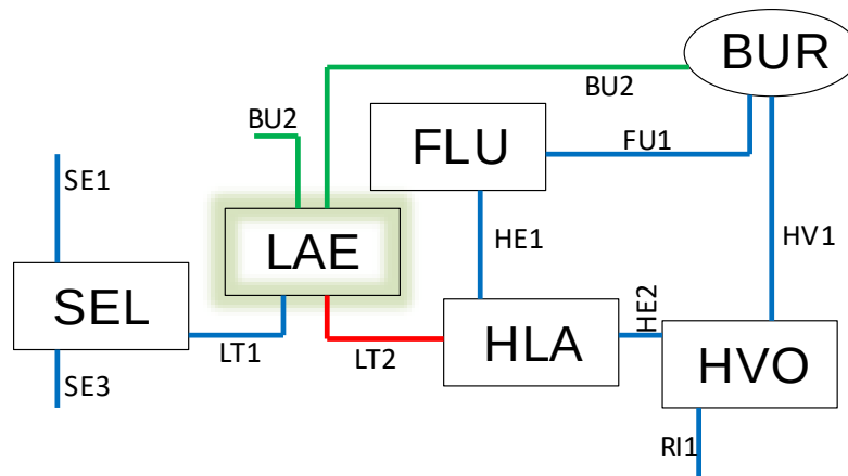
MYND 3-33 : EINLÍNUMYND AF FLUTNINGSKERFINU Á SUÐURLANDI MEÐ NÝJU TENGIVIRKI VIÐ LÆKJARTÚN
