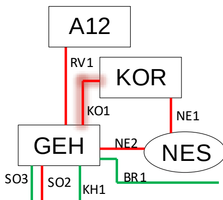
MYND 3-40 : EINLÍNUMYND KORPULÍNU 1
