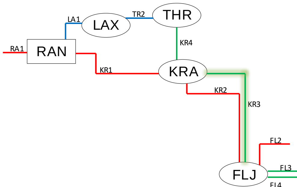
MYND 3-3 : EINLÍNUMMYND KRÖFLULÍNU 3, Í MEGINDRÁTTUM MEÐFRAM KRÖFLULÍNU 2
