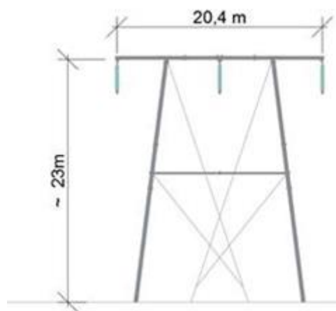
MYND 3-59: STAGAÐ STÁLÖRAMASTUR AF M-GERÐ
